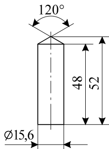
Abb. 2: Zylindrischer Bronzekolben; Masse in mm
