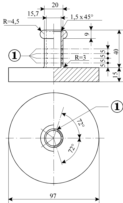
Abb. 3: Hohler Bronzezylinder, einseitig verschlossen Aufriss und Grundriss; Masse in mm
